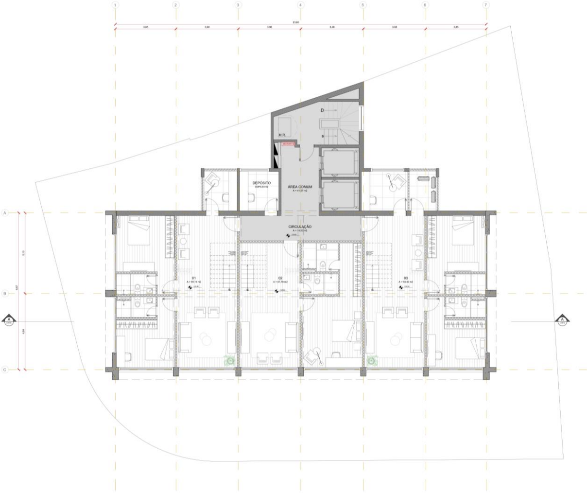
proposta | escala 1:75
