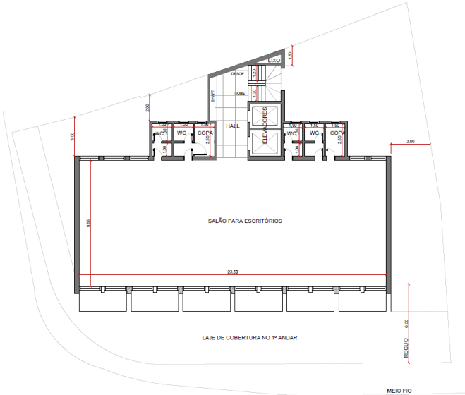
situação atual
