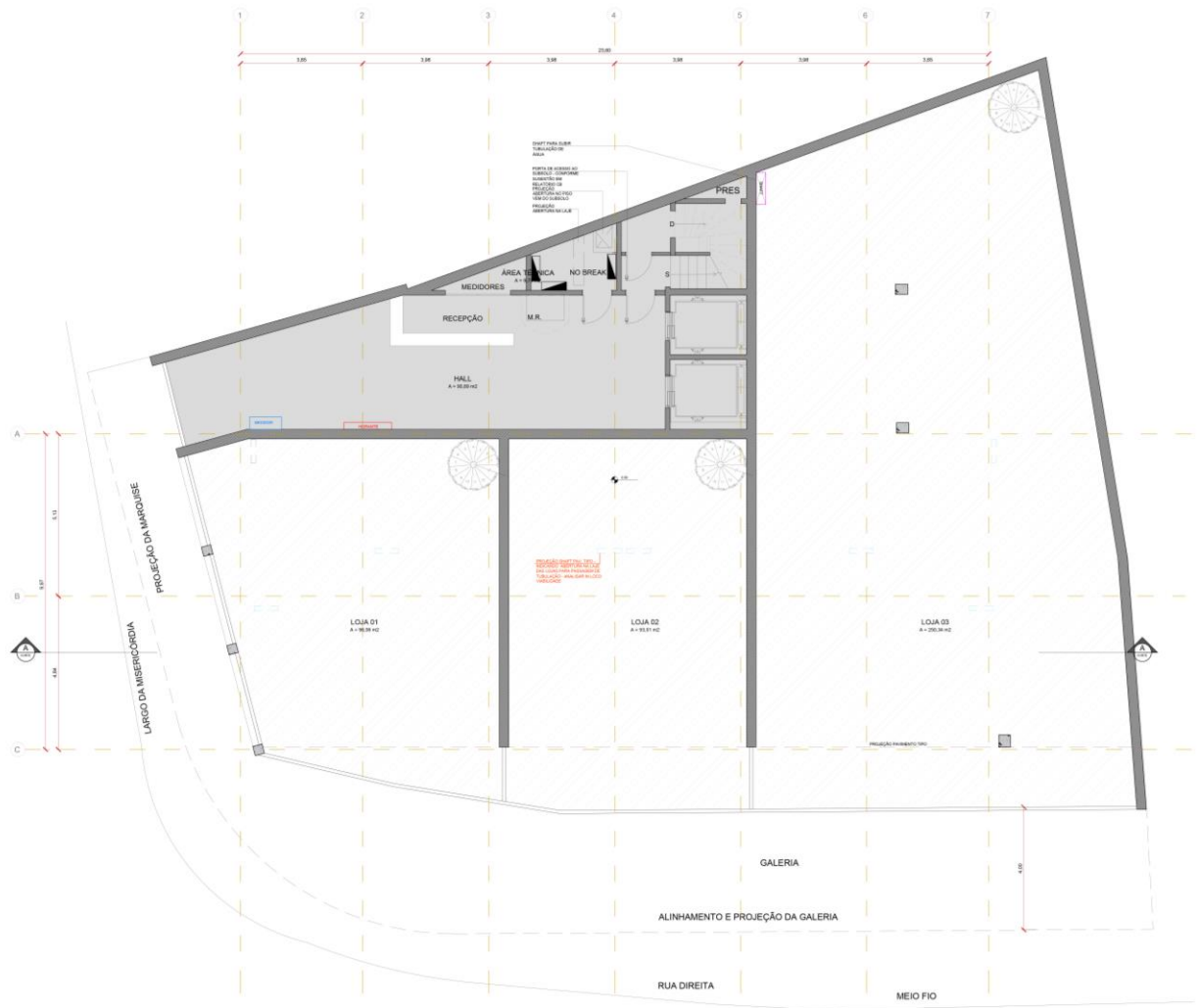
proposta | escala 1:75
