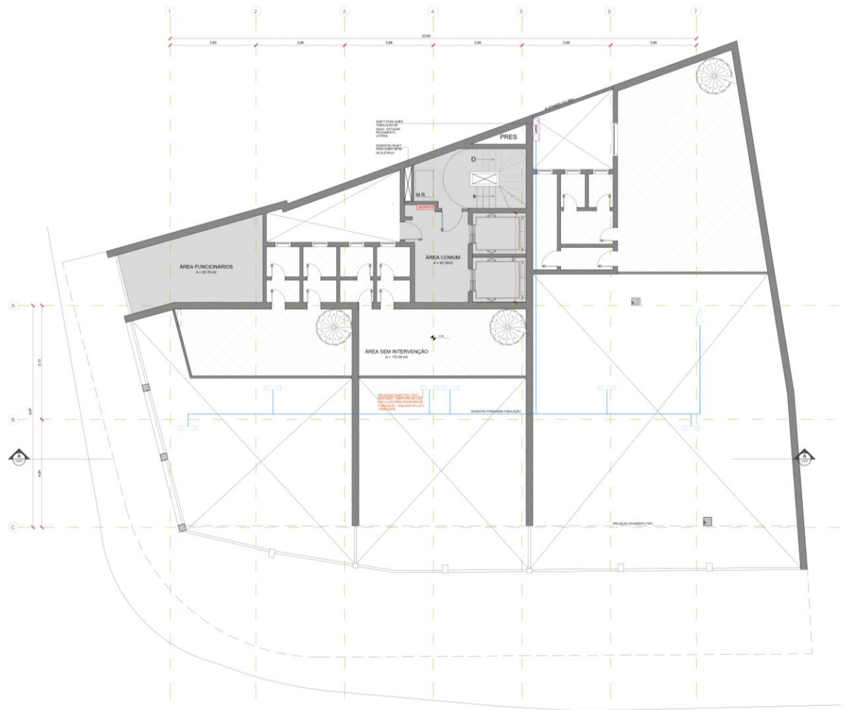
proposta | escala 1:75
